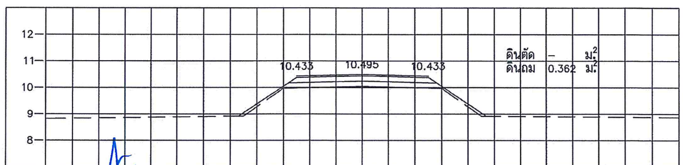
STA. 0+575.000 NGL = 10.025
