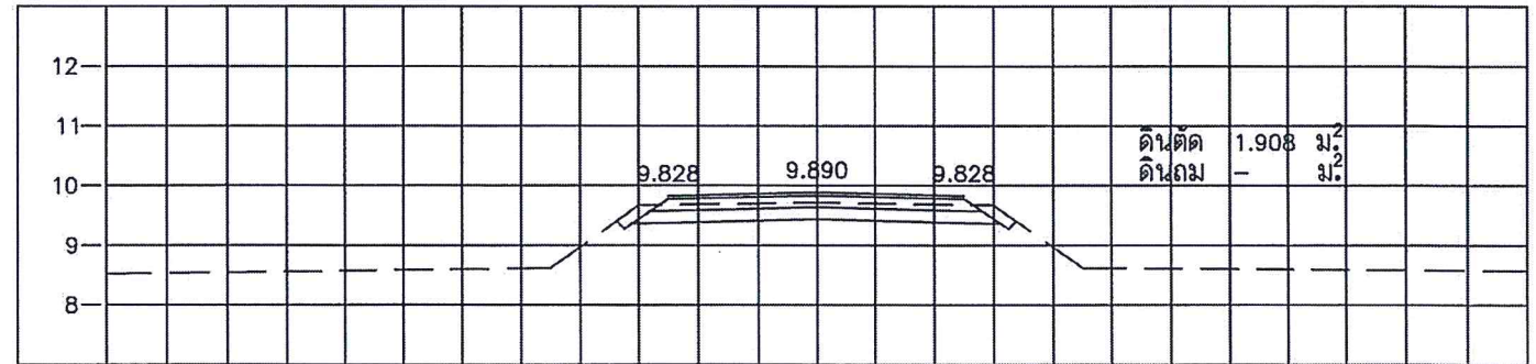
STA. 0+175.000 NGL = 9.721
