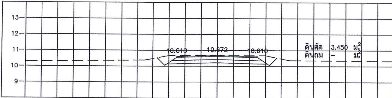
STA. 1+175.000 NGL = 10.672
