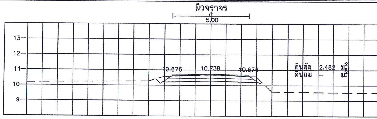
STA. 1+675.000 NGL = 10.678
