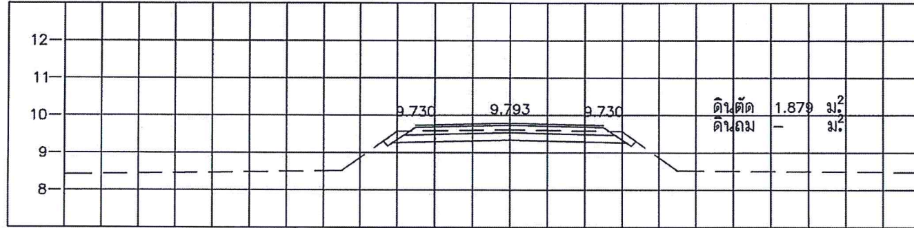
STA. 0+075.000 NGL = 9.619
