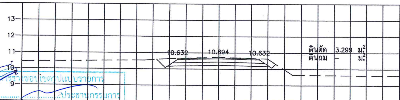
STA. 1+575.000 NGL = 10.739
