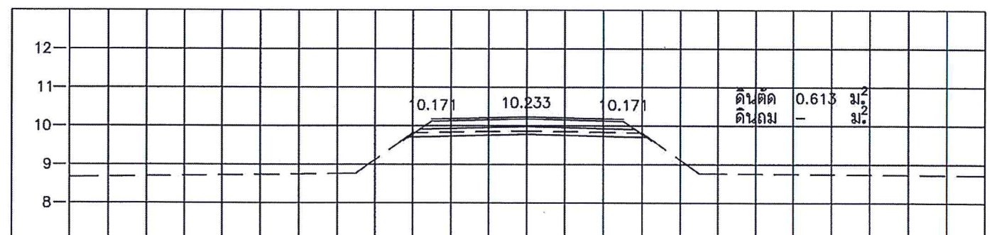
STA. 0+400.000 NGL = 9.869
