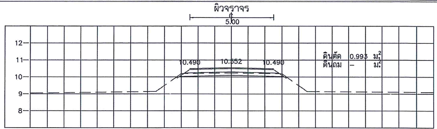
STA. 0+650.000 NGL = 10.246
