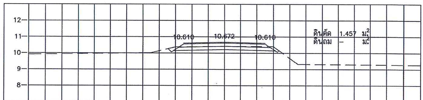
STA. 1+275.000 NGL = 10.417
