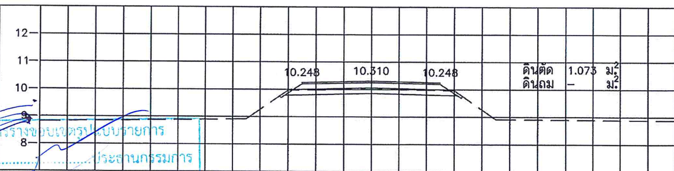
STA. 0+450.000 NGL = 10.016
