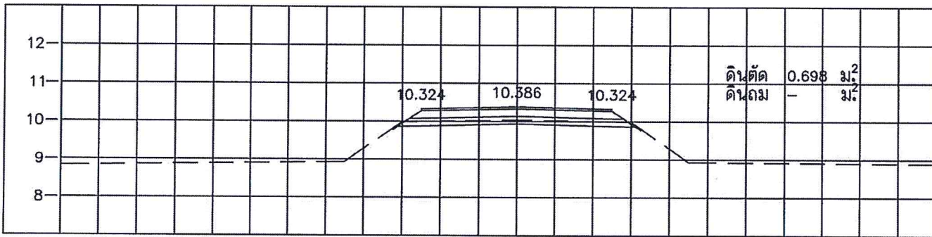
STA. 0+500.000 NGL = 10.035
