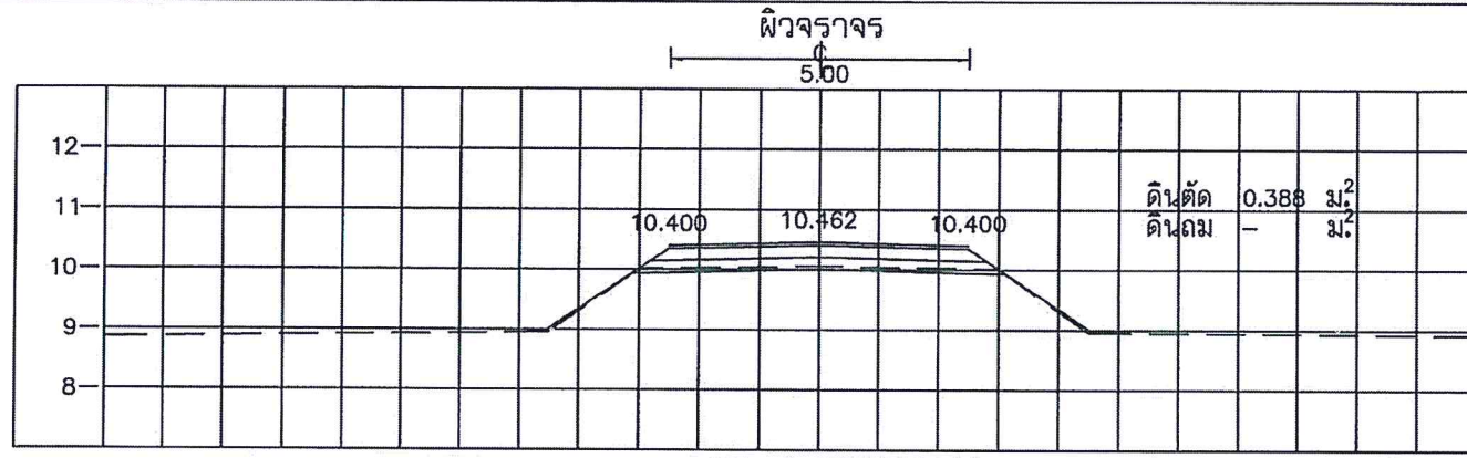
STA. 0+550.000 NGL = 10.063
