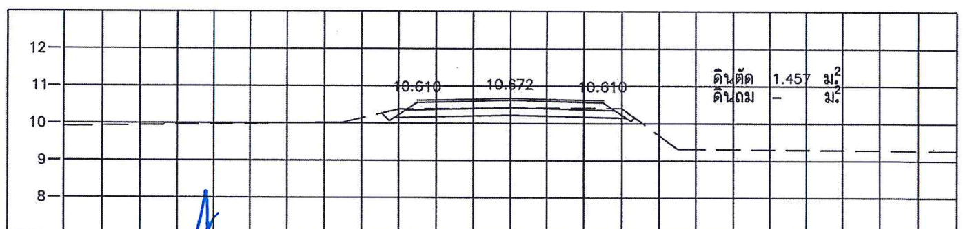
STA. 1+250.000 NGL = 10.417
