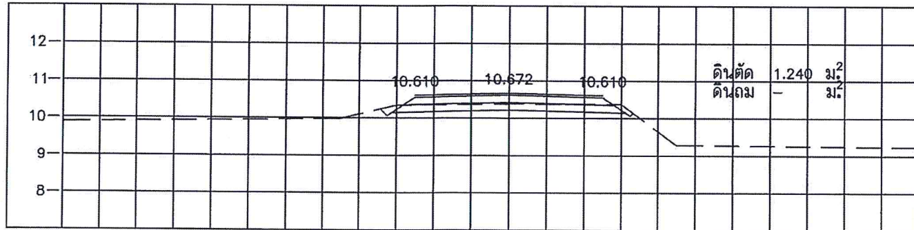
STA. 1+200.000 NGL = 10.385
