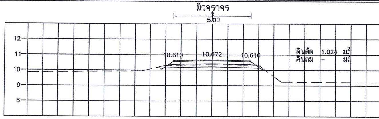
STA. 1+225.000 NGL = 10.353
