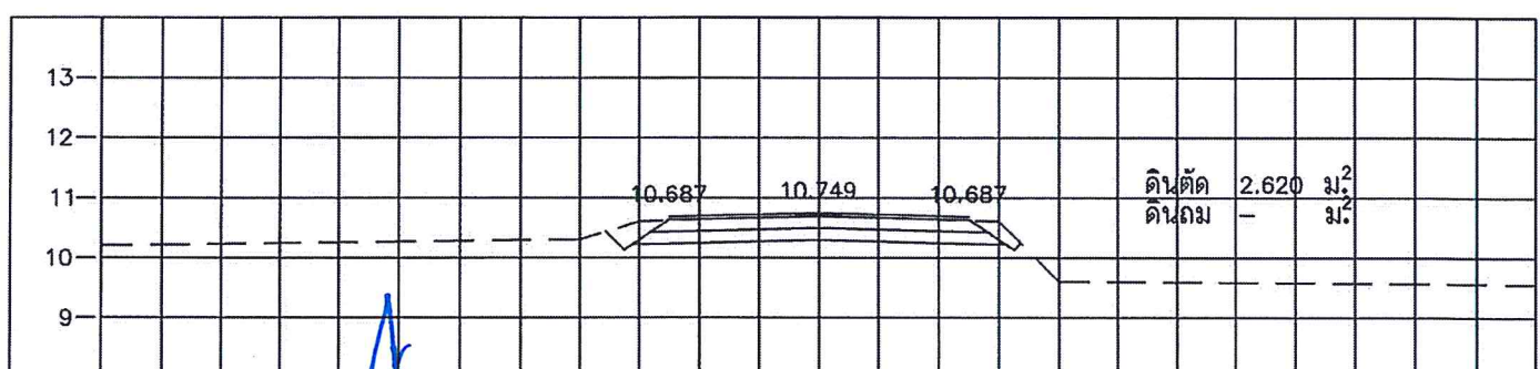
STA. 1+700.000 NGL = 10.709
