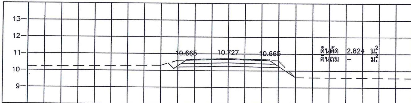
STA. 1+650.000 NGL = 10.706
