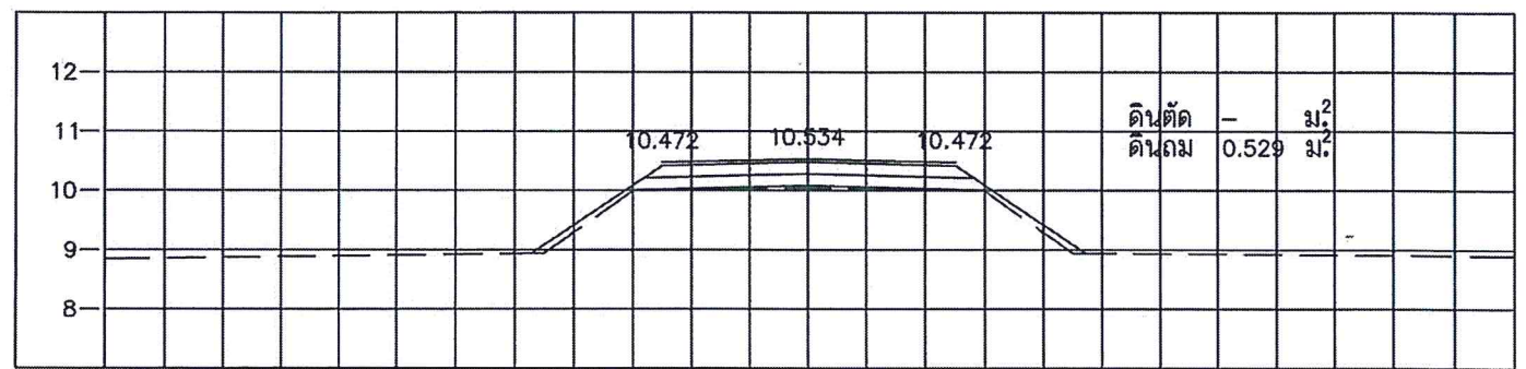
STA. 0+625.000 NGL = 10.046
