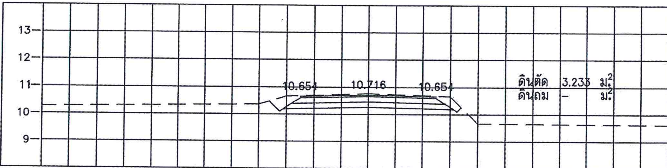
STA. 1+625.000 NGL = 10.764
