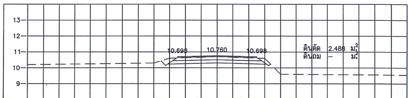
STA. 1+725.000 NGL = 10.701
