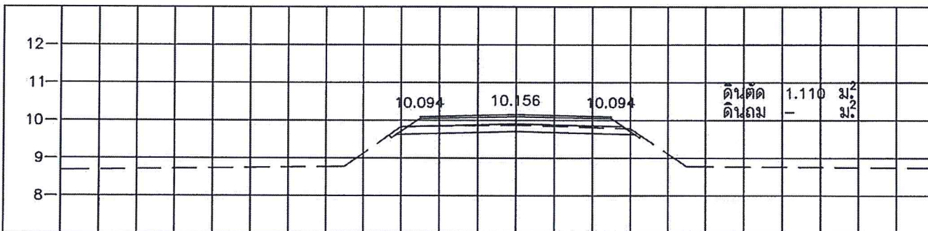
STA. 0+025.000 NGL = 9.881
