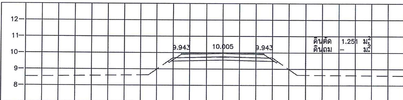
STA. 0+250.000 NGL = 9.738
