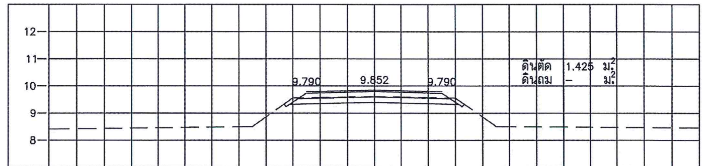
STA. 0+150.000 NGL = 9.611
