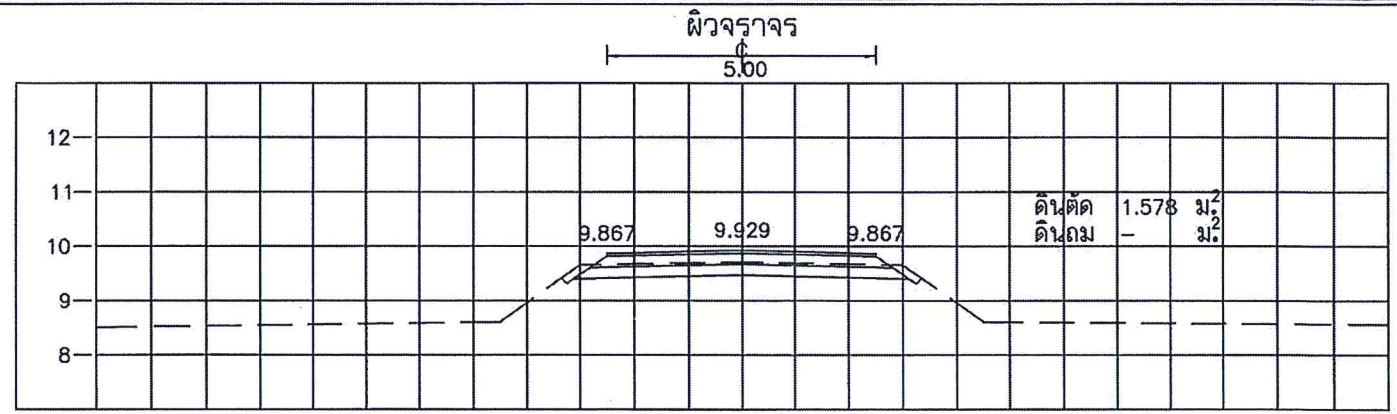
STA. 0+200.000 NGL = 9.711
