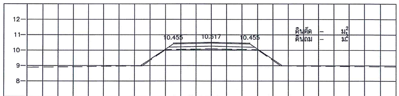
STA. 0+600.000 NGL = 10.090
