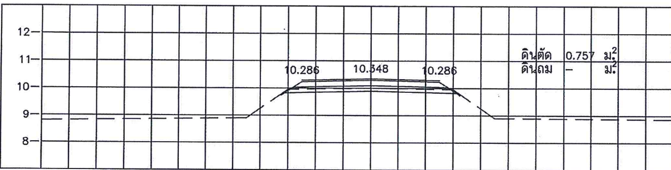
STA. 0+475.000 NGL = 10.006
