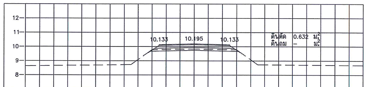
STA. 0+375.000 NGL = 9.834
