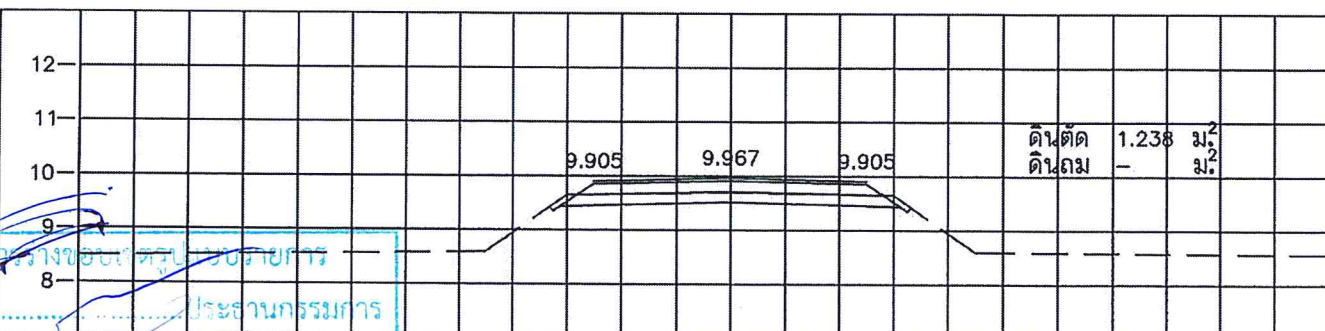
STA. 0+225.000 NGL = 9.698
