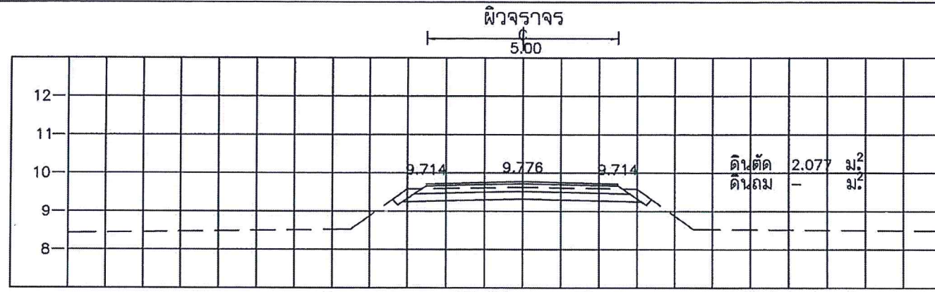
STA. 0+100.000 NGL = 9.632
