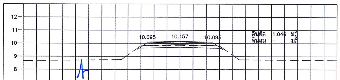
STA. 0+350.000 NGL = 9.859
