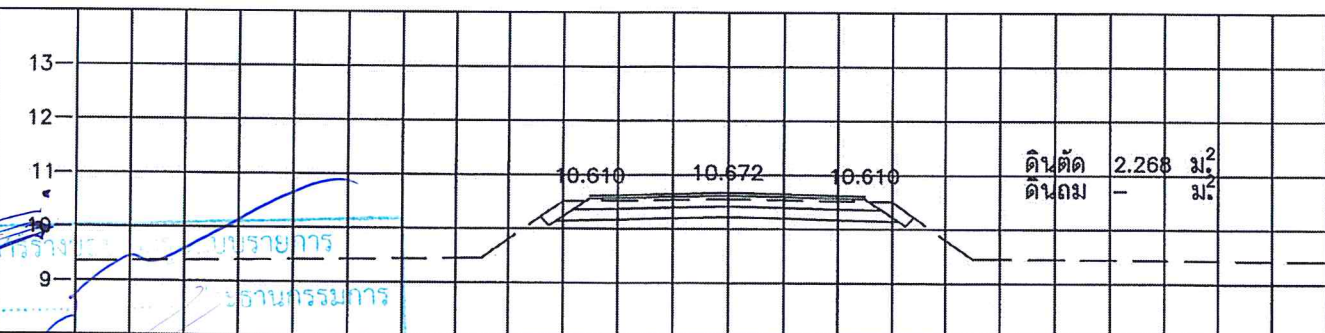
STA. 1+125.000 NGL = 10.556
