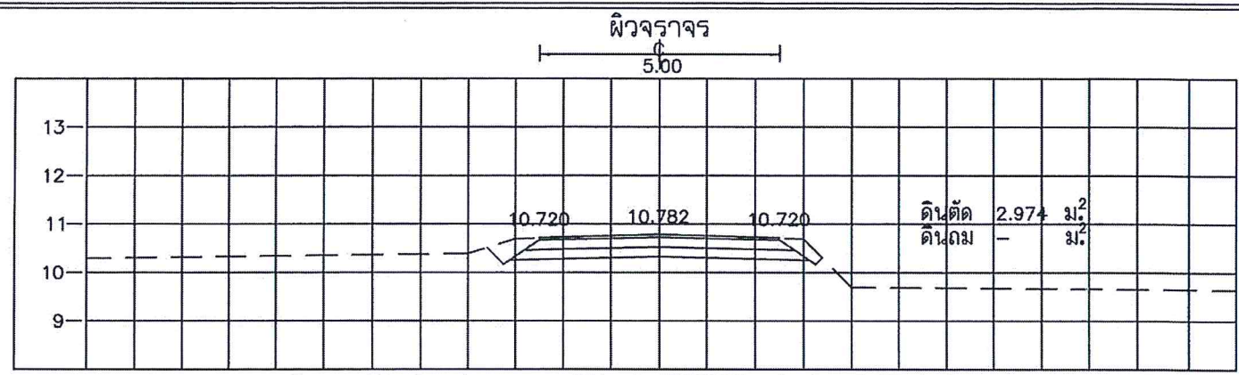
STA. 1+775.000 NGL = 10.793
