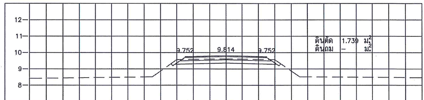
STA. 0+125.000 NGL = 9.620
