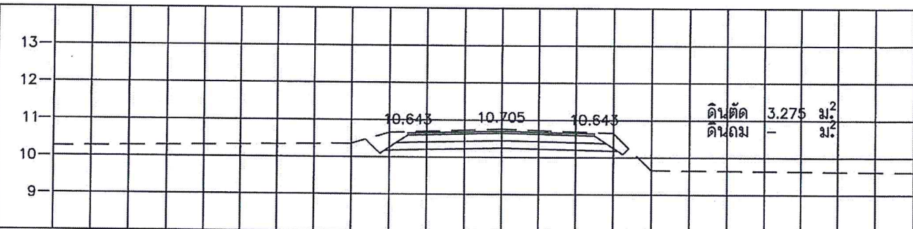
STA. 1+600.000 NGL = 10.759
