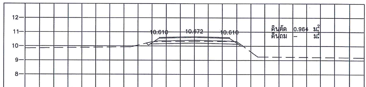
STA. 1+300.000 NGL = 10.344
