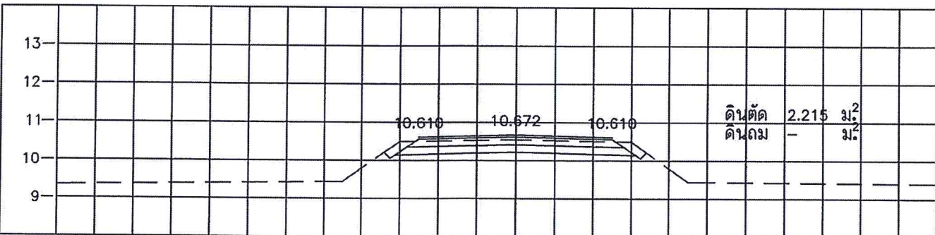
STA. 1+150.000 NGL = 10.550
