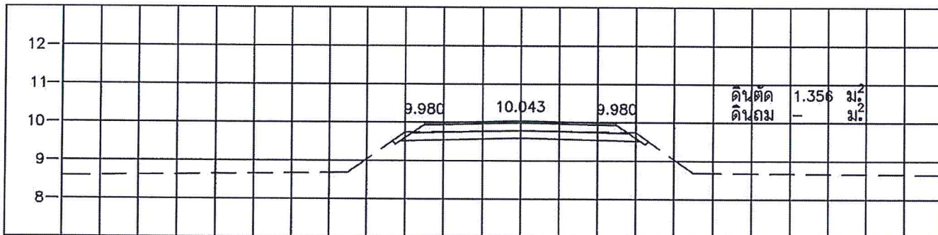
STA. 0+275.000 NGL = 9.791
