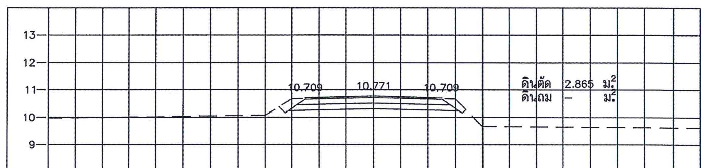
STA. 1+750.000 NGL = 10.774
