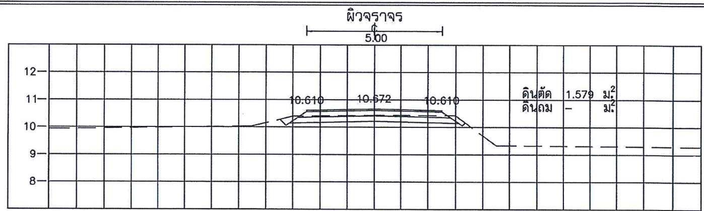
STA. 1+325.000 NGL = 10.435
