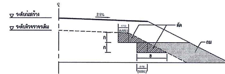
รูปตัดการก่อสร้างลาดคันทาง
