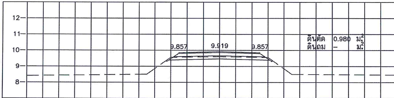
STA. 0+050.000 NGL = 9.611
