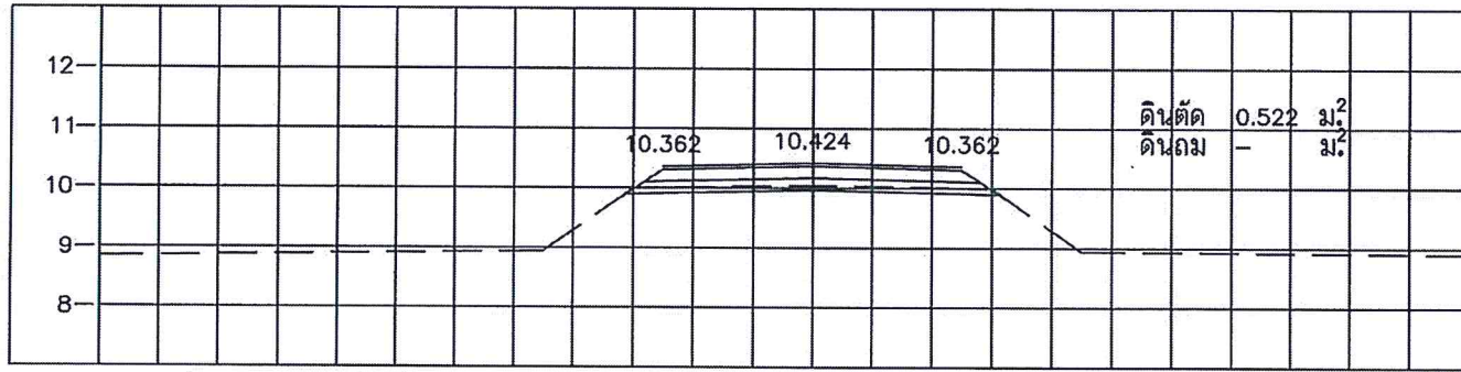
STA. 0+525.000 NGL = 10.046
