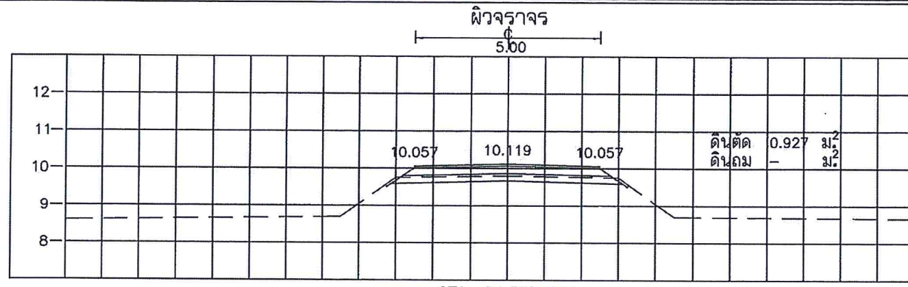
STA. 0+325.000 NGL = 9.803
