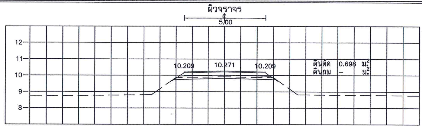
STA. 0+425.000 NGL = 9.920
